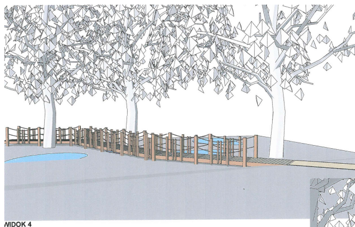
Ryc. 6. Projekt ścieżka przez bagna w dolinie Cybiny
